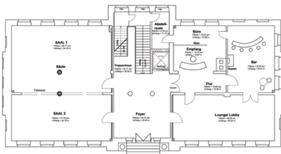
Grundriss Prinzenpalais EG
